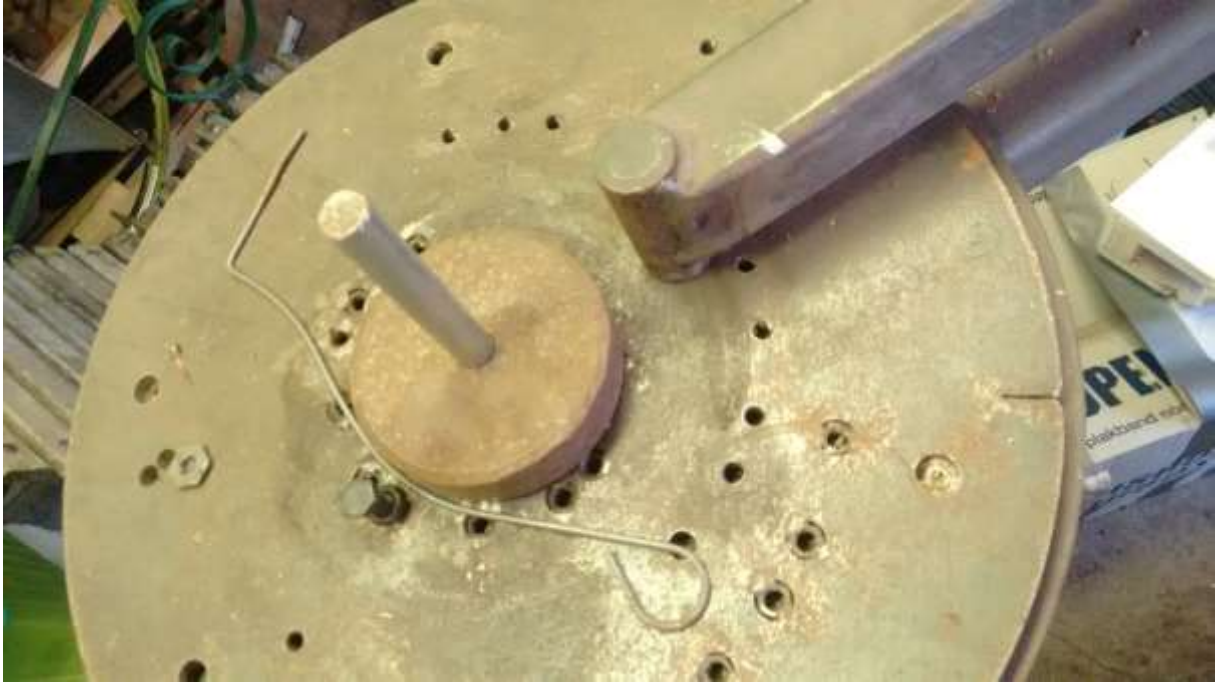
Buigapparaat.verschillende rondingen kunnen gemonteerd worden voor verschillende buigingen van het materiaal zie voorbeeld .
